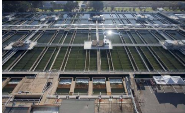
Deler av vannbehandlingsanlegget ved elven Ter, sett fra høyden
